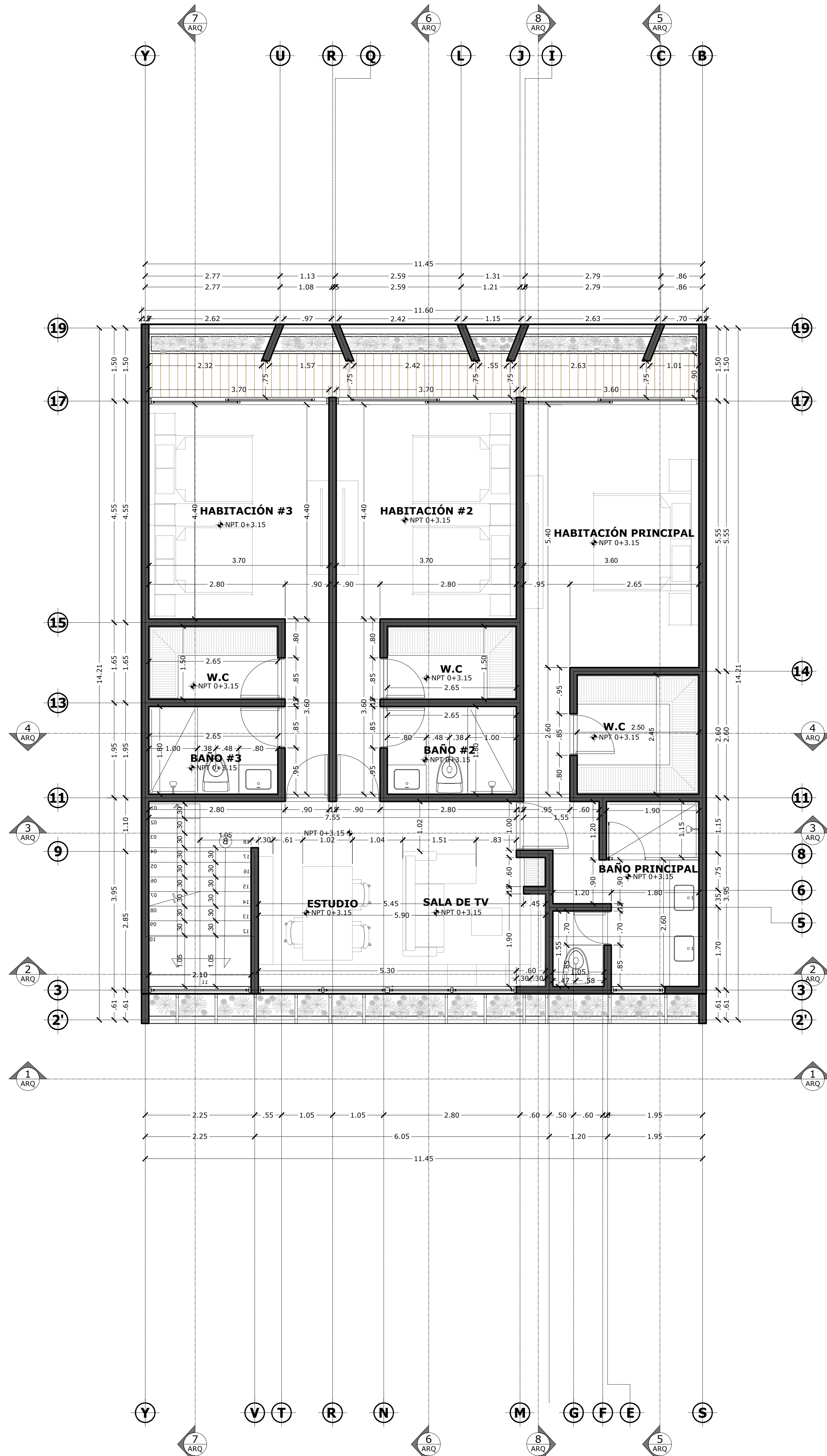
PLANTA ARQUITECTÓNICA NIVEL 2 ACQUARELLO ALTO DE LAS PALOMAS CASA DE HABITACIÓN
