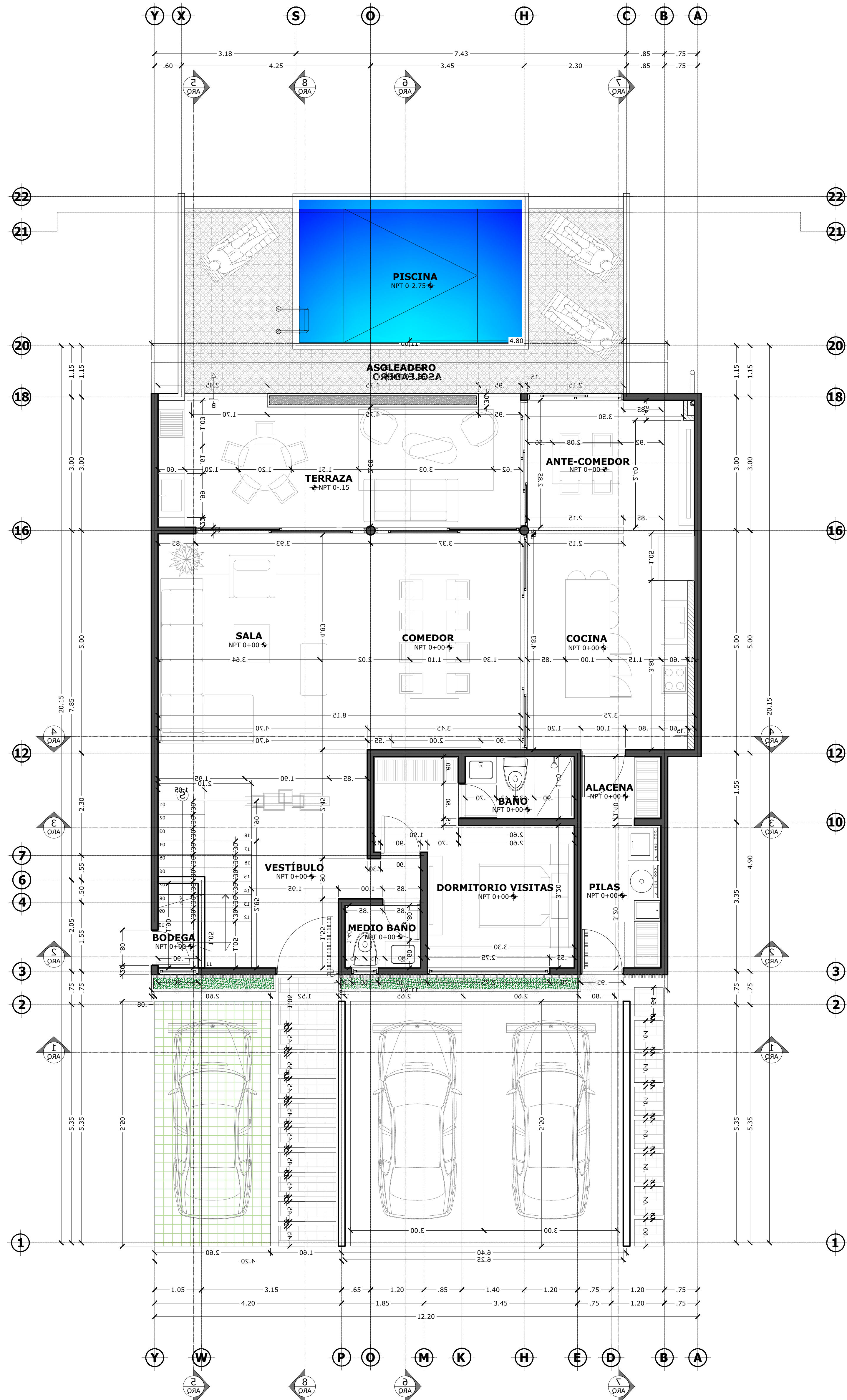
PLANTA ARQUITECTÓNICA NIVEL 1 ACQUARELLO ALTO DE LAS PALOMAS CASA DE HABITACIÓN
