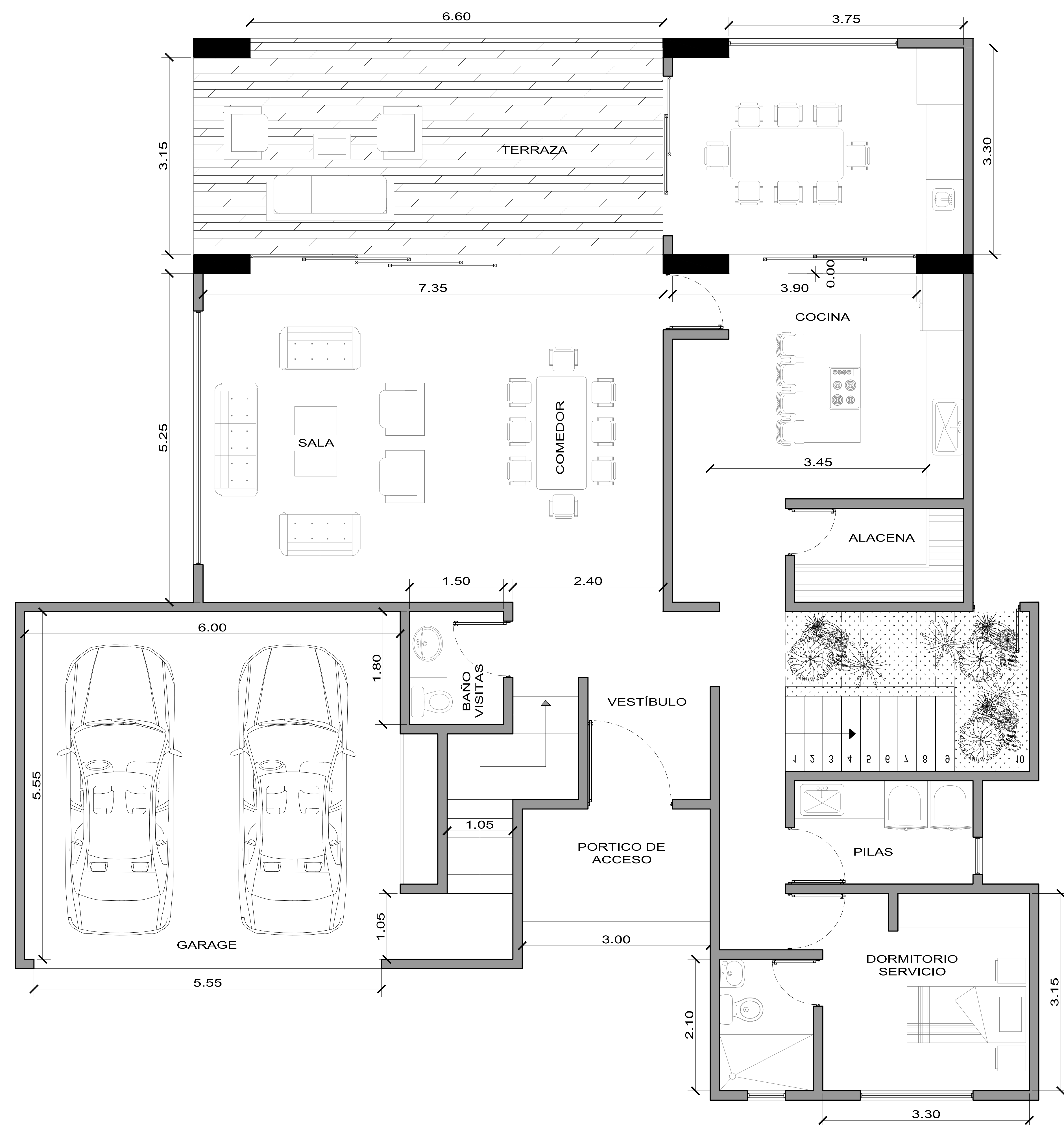
PLANTA DE DISTRIBUCIÓN ARQUITECTÓNICA PRIMER NIVEL 215M2
