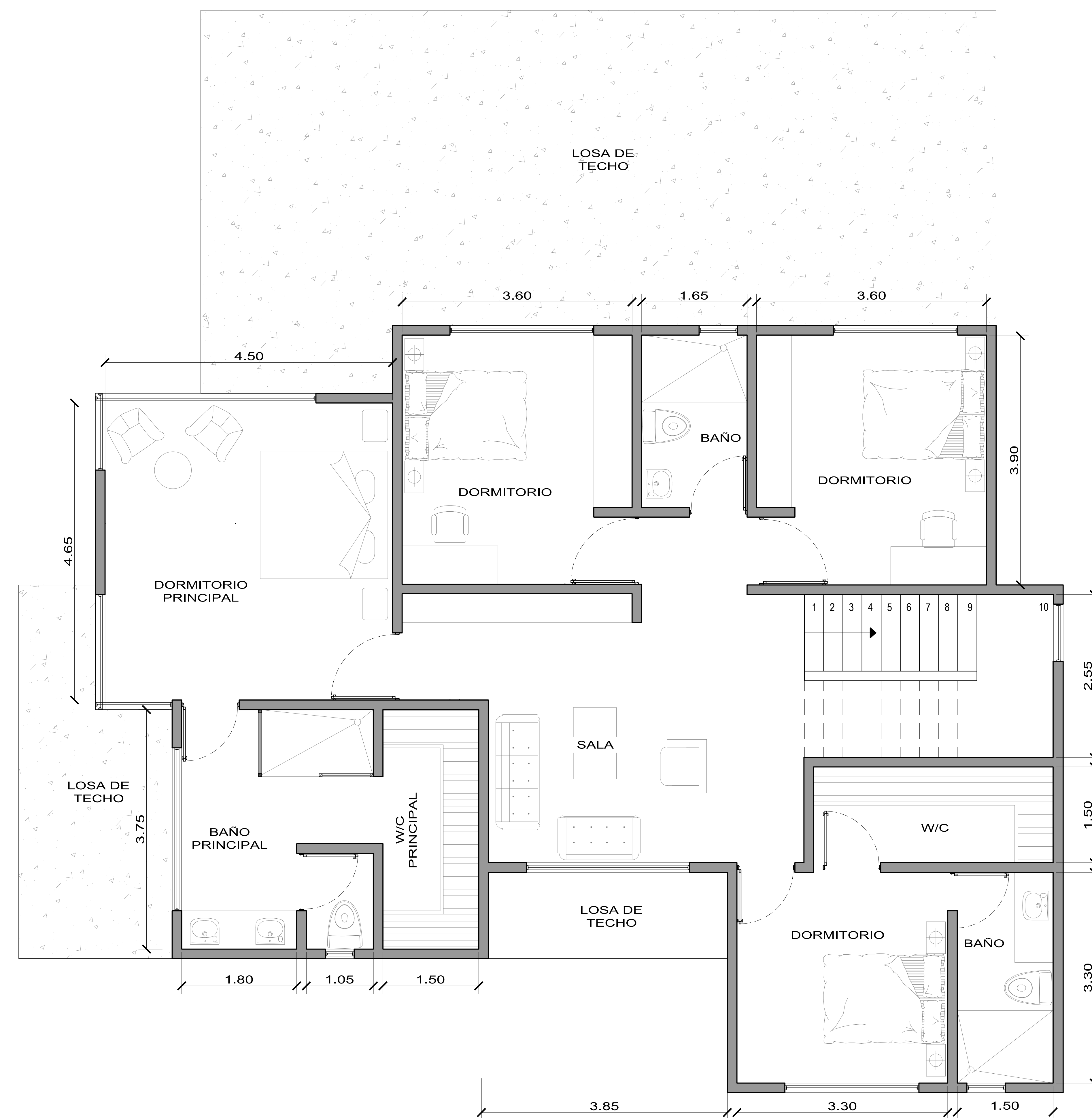
PLANTA DE DISTRIBUCIÓN ARQUITECTÓNICA SEGUNDO NIVEL ÁREA:142M2 (SIN LOSAS DE TECHO NI BALCONES)
