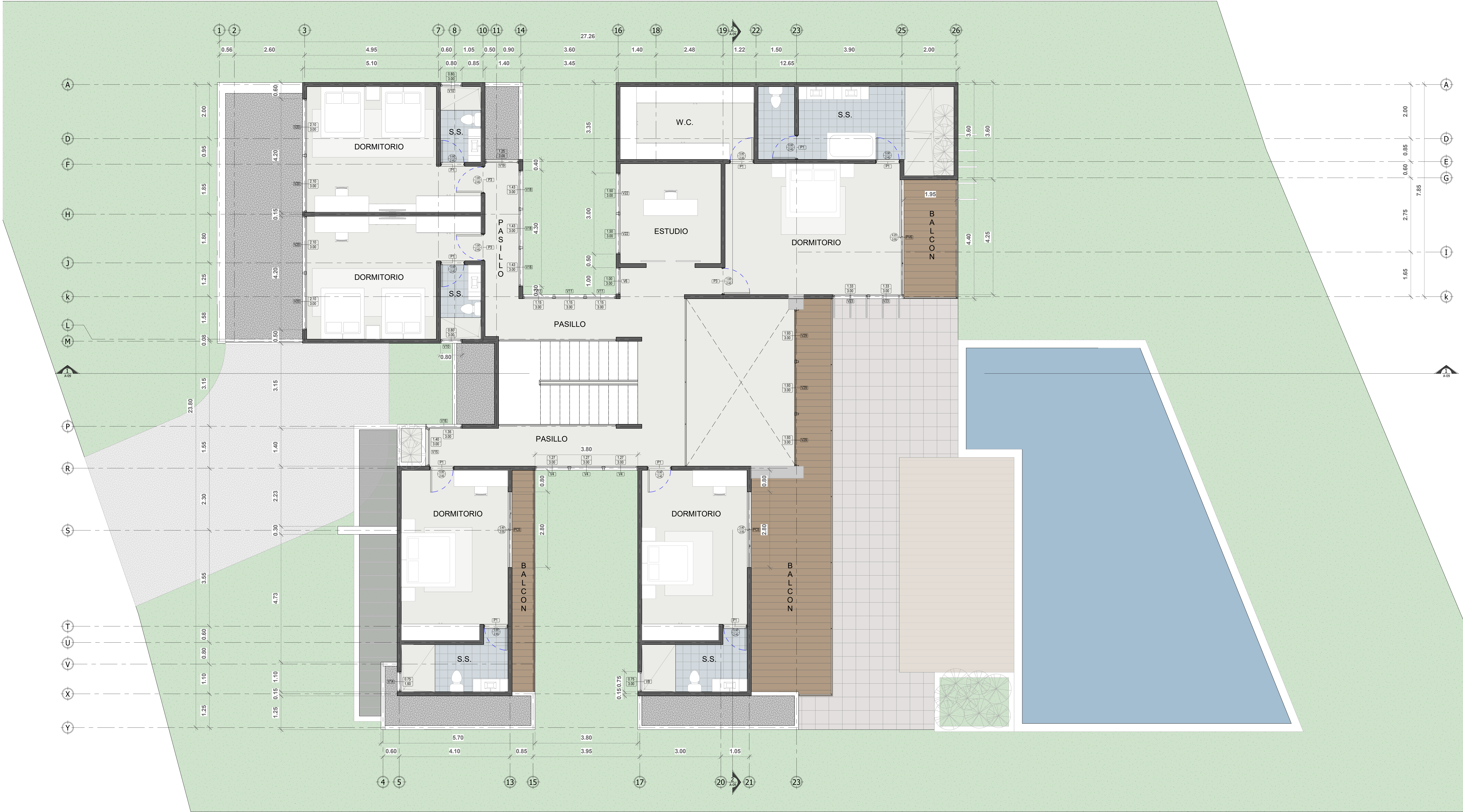
1 PLANTA ARQUITECTONICA 2 NIVEL 1 : 50
