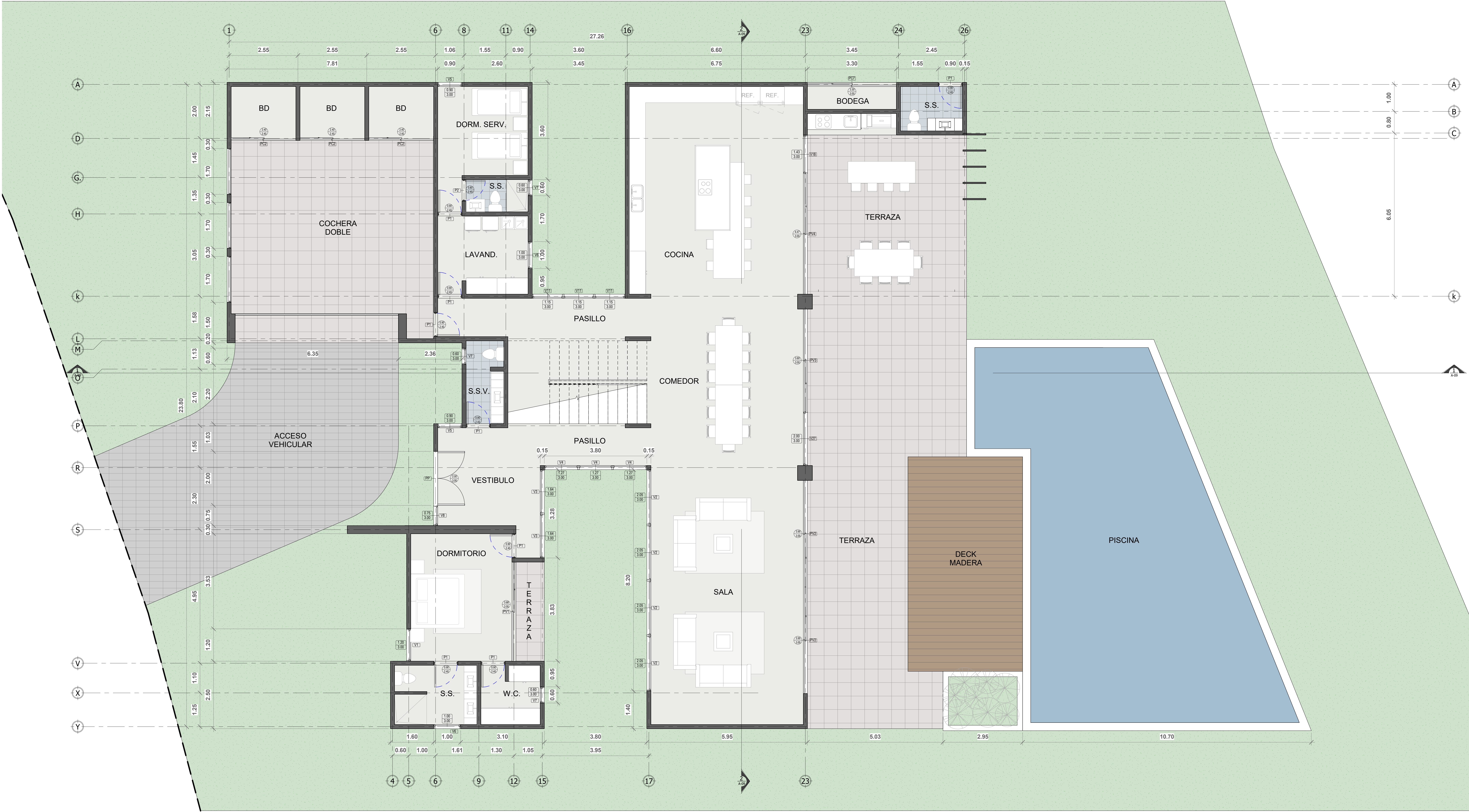
1 PLANTA ARQUITECTONICA 1 NIVEL 1 : 50
