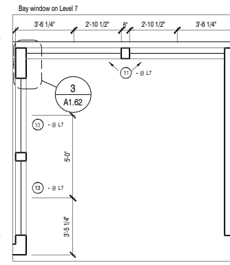
3 Unit type E A502 SCALE: 1/4" = 1'-0" 1/8" = 1'-0"
