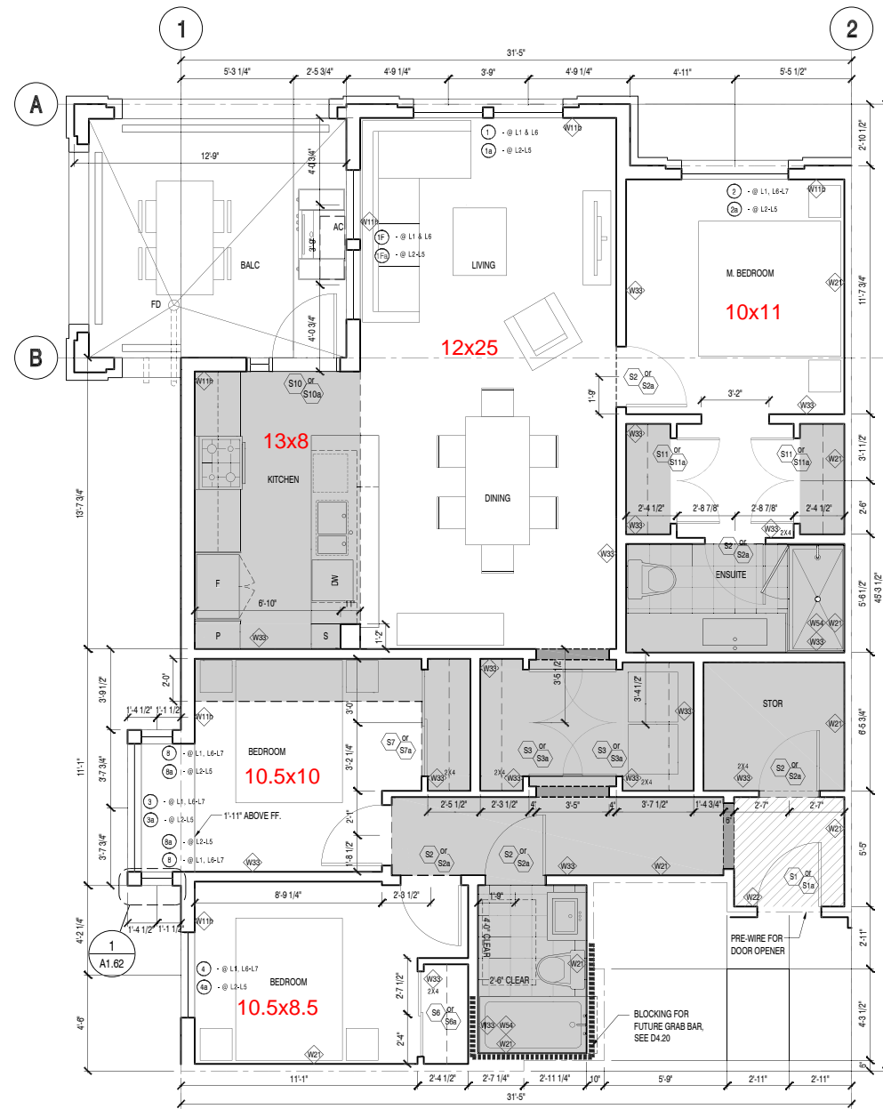
3 Unit type E A502 SCALE: 1/4" = 1'-0" 1/8" = 1'-0"
