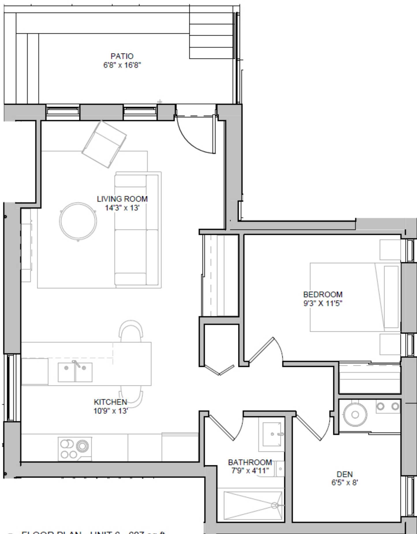
① FLOOR PLAN - UNIT 6 - 607 sq ft 1 : 48
