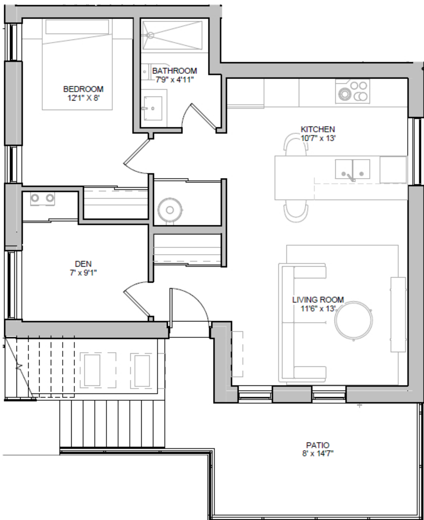
① FLOOR PLAN - UNIT 3 - 571 sq ft 1 : 48
